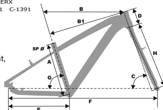
GEOMETRIE RÁMU 24" MRX X7
